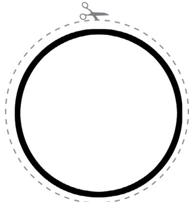
Jupiter
