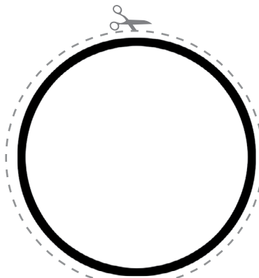
Uranus
